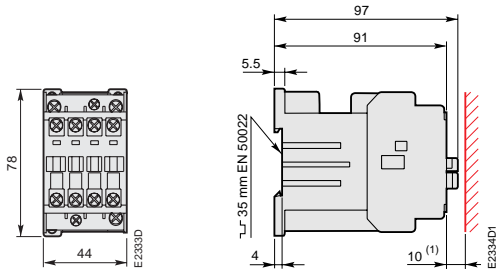
AL 9 ... AL 16, AL..Z. TAL 9 ... TAL 16 NL., NL Z., TNL..
